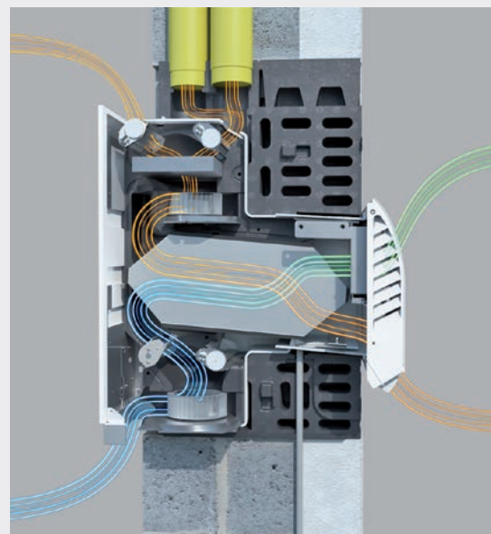
Querschnitt freeAir 100 mit Gegenstrom-Wärmetauscher
